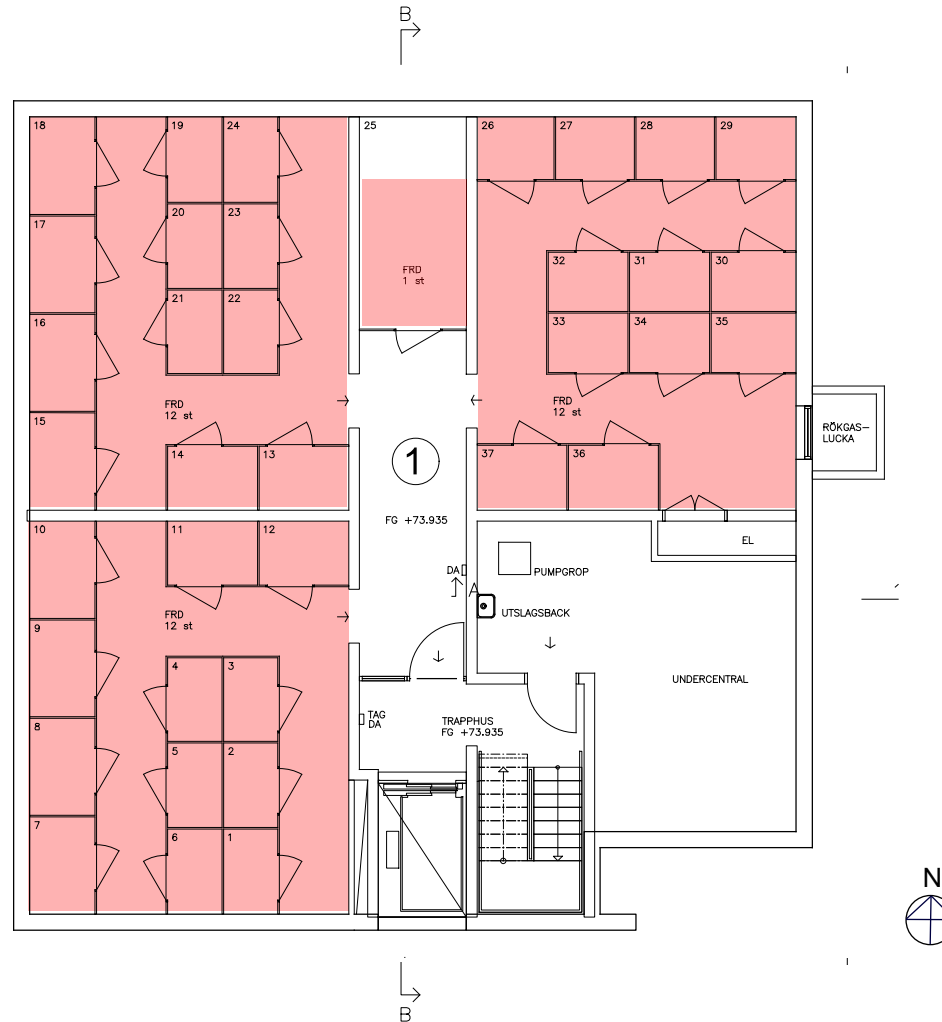
PLAN 09, KÄLLARPLAN
