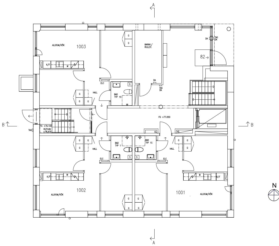
PLAN 10, ENTRÉPLAN
